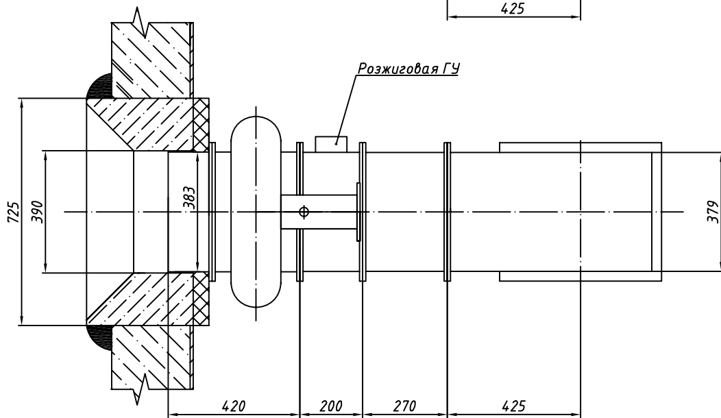
Котел КВГМ-10
