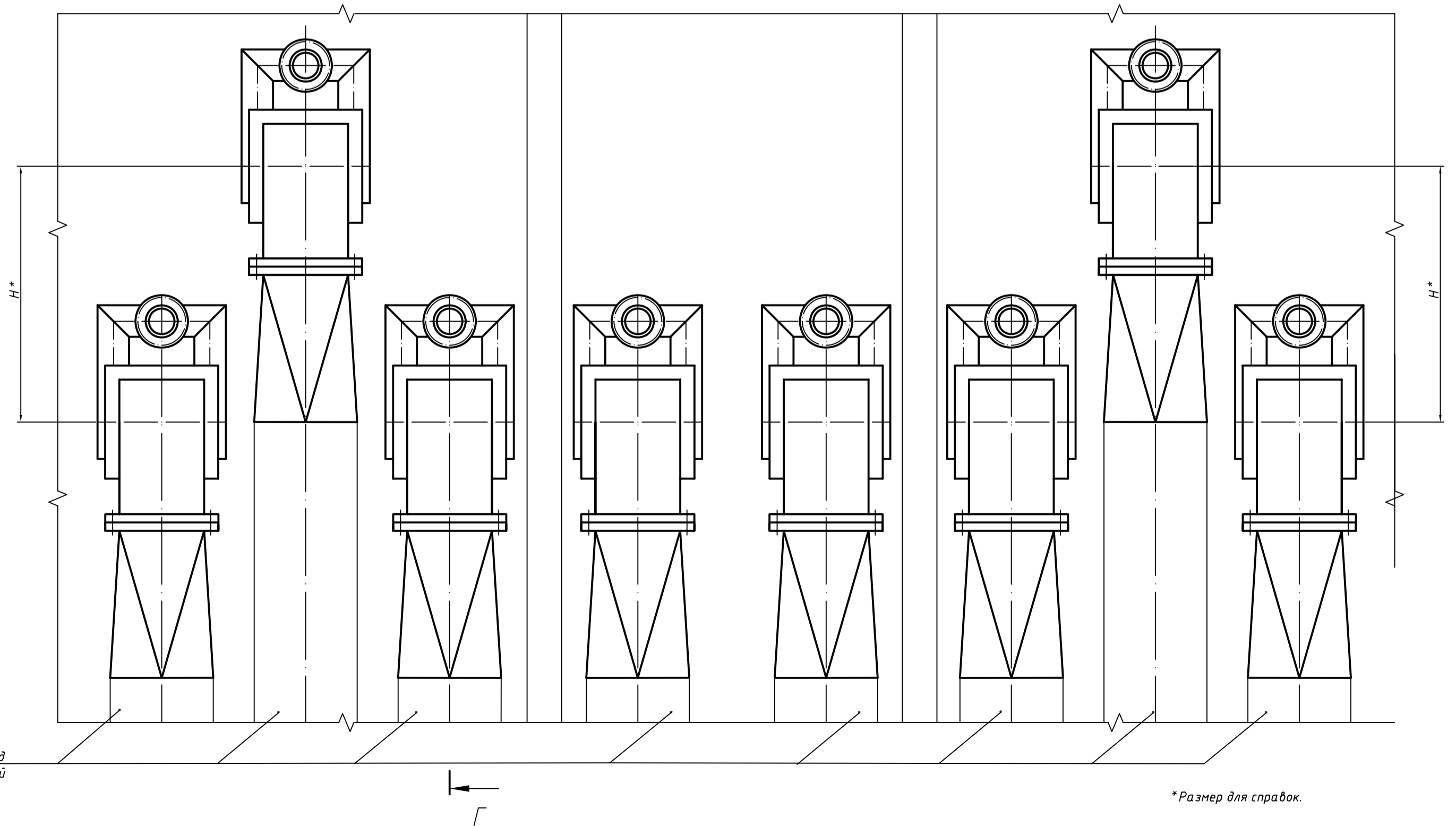
Котел ПТВМ-100 с шестнадцатью горелками
